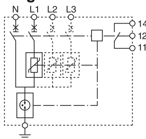
1P+N / 3P+N.
